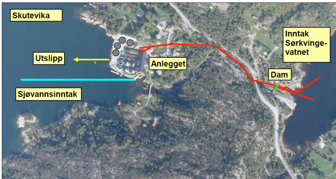
Figur 1. Oversikt over smoltanlegget på Kvinge med tilhørende rørgater for inntak av ferskvann fra Sørkvingevatnet, dammen ved utløpet av Sørkvingevatnet, utslippene samt sjøvannsinntaket i Skutevika.
